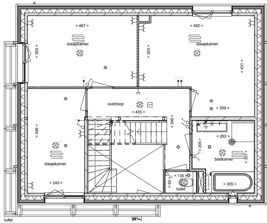
eerste verdieping
