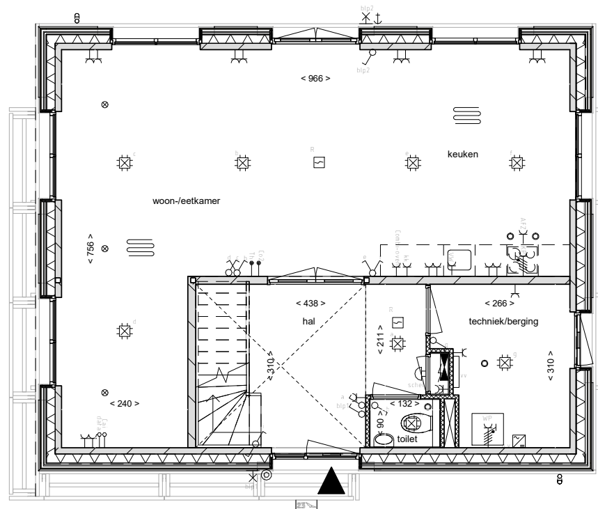
begane grond
